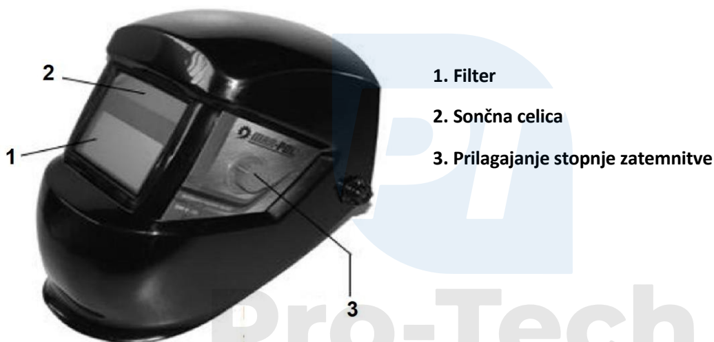
Opis filtra
